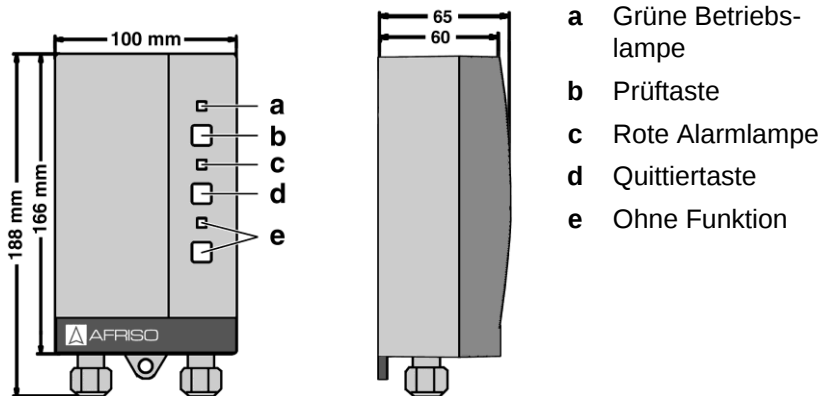
Bild 2: Steuergerät
