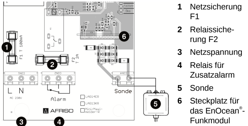
Bild 6: Elektrischer Anschluss
