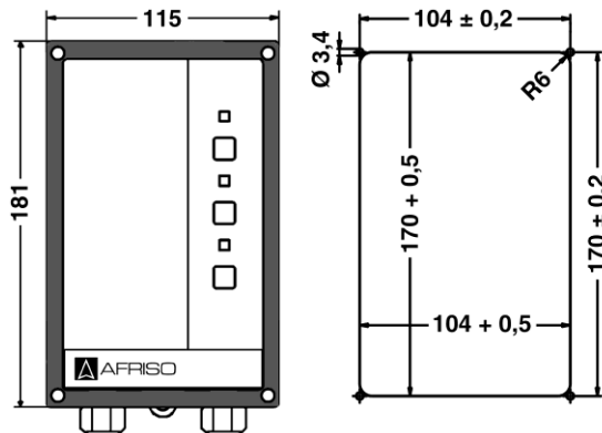
Bild 5: Steuergerät mit Montagerahmen für den Einbau in Schalttafeln; rechts: Schalttafelausschnitt
