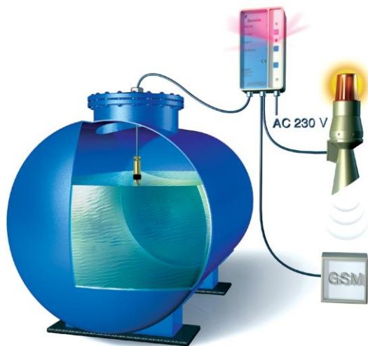
Bild 4: Standardanwendung Maximelder-R
