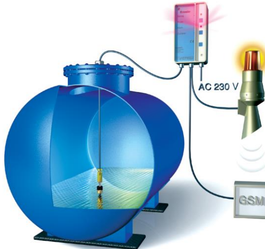
Bild 3: Standardanwendung Minimelder-R
