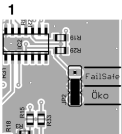
Bild 7: Jumper
