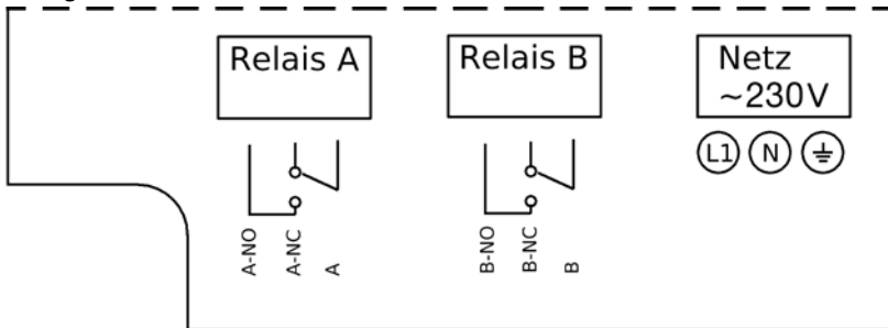
Bild 6: Anschlussplan
